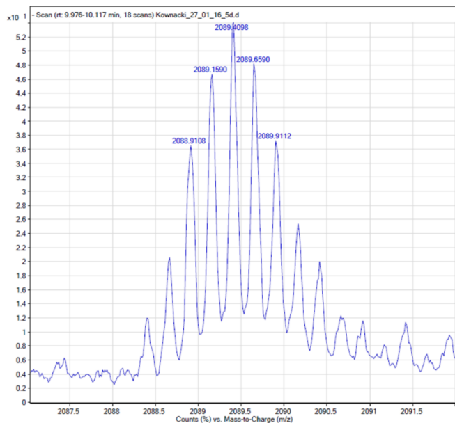
Figure 49. ESI-MS analysis of oligomer N.
